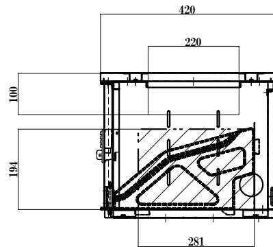
【右側面図】
