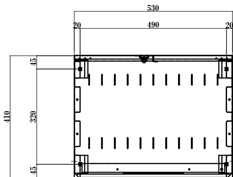
【底面図】
