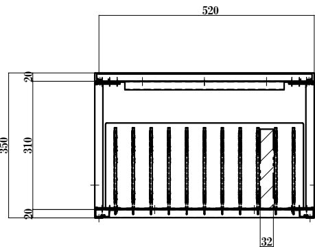
【正面断面図】
